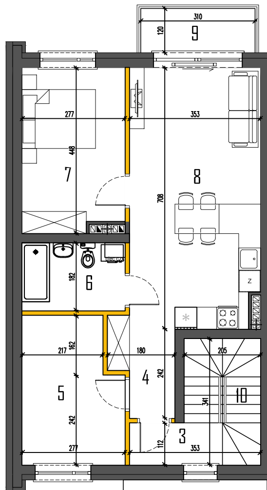
RZUT PIĘTRA
