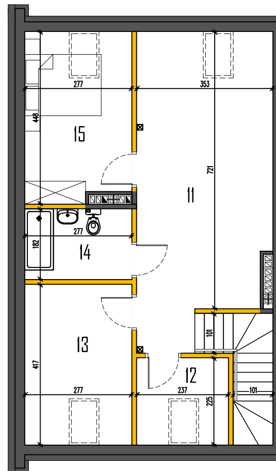
RZUT PODDASZA
